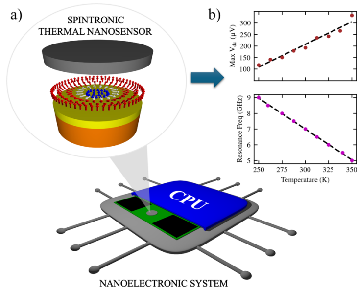
Figura 1: a) Rappresentazione schematica del dispositivo proposto, b) Andamento lineare dell'ampiezza massima della tensione di rettificazione ( V_{dc,max} ) e della frequenza di risonanza ( \omega_F ) con la temperatura per il dispositivo Single FL MTJ.
