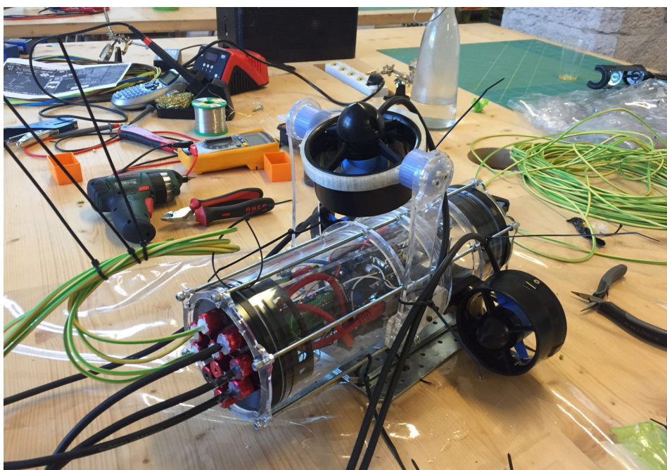
Fig. 2: Prototipo di ArcheoROV
